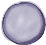
RegExp
